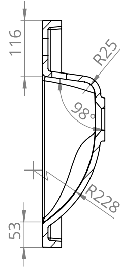
PRZEKRÓJ M-M SKALA 1 : 8
