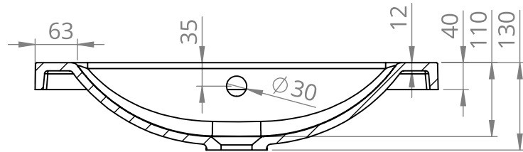
PRZEKRÓJ N-N SKALA 1 : 8
